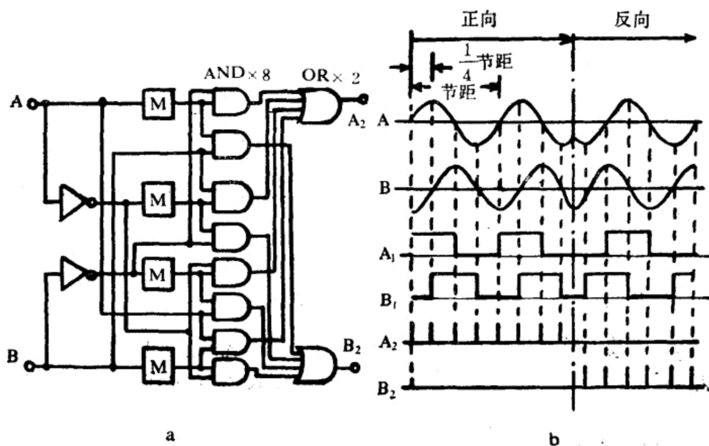
图 3.8.8 零点基准法
