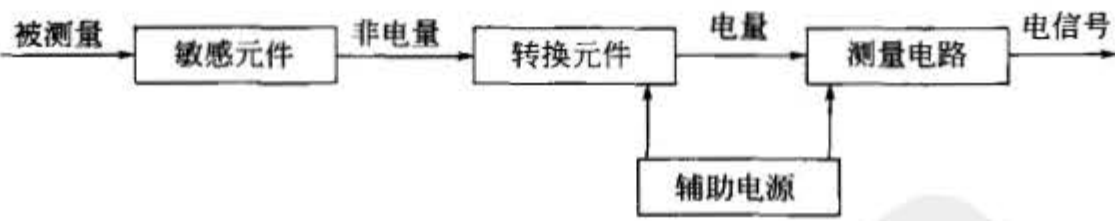
图 1-3 传感器组成框图
